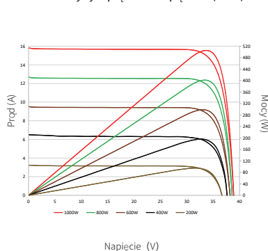
Charakterystyka prądowo - napięciowa (500W)
